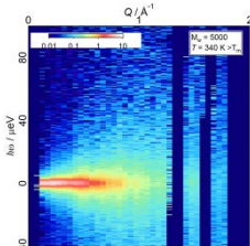
高分子鎖のダイナミクスの測定
