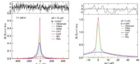
吸着水と自由水を区別したダイナミクスの測定
