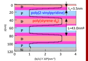
中性子反射率データの解析結果。軽水素・重水素化ポリマーの違いが散乱長密度の差として明確に現れている。
